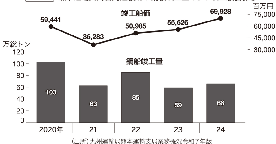
グラフ1 熊本運輸支局管内造船所の鋼船竣工量および竣工船価推移
